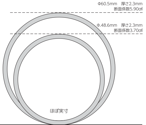
大型防球ネット バッティングケージ等に採用
