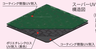
UVシート 構造図
